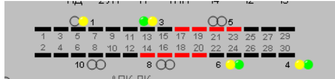
Рис.296. Схематичное изображение перегона между станциями на мнемосхеме
