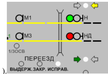
Рис.293. Изображение переезда на мнемосхеме станции
