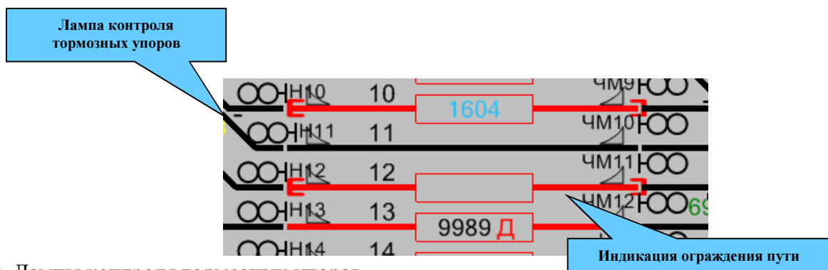
Рис.292. Лампы контроля тормозных упоров
